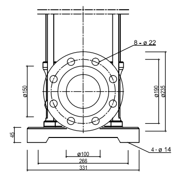
F(DIN) PN 25-40 (DN100) /mm/
