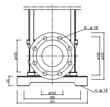
F(DIN) PN16 (DN100) /mm/
