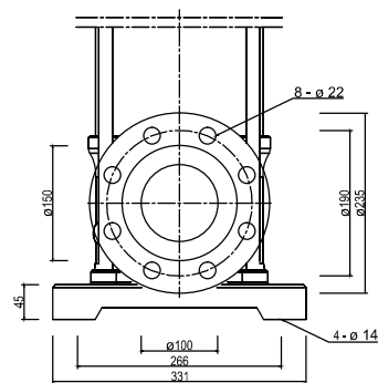
F(DIN) PN 25-40 (DN100) /mm/
