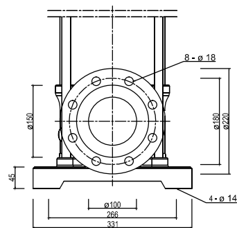
F(DIN) PN16 (DN100) /mm/
