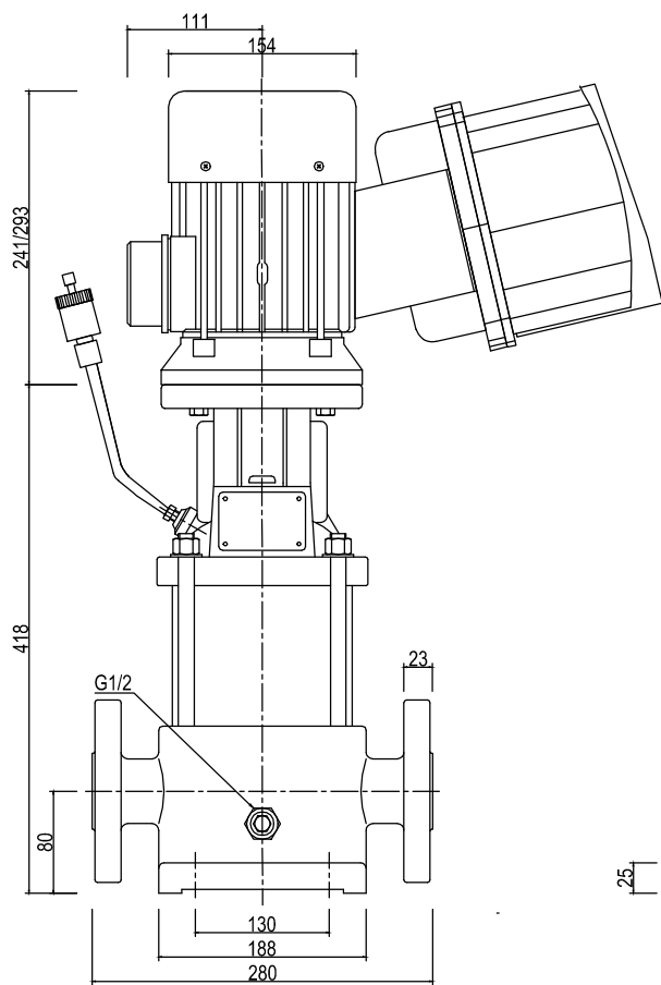
FGJ(DIN-ANSI-JIS) PN25(DN40) /mm/
