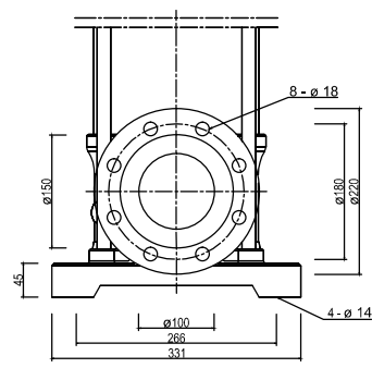
F(DIN) PN16 (DN100) /mm/
