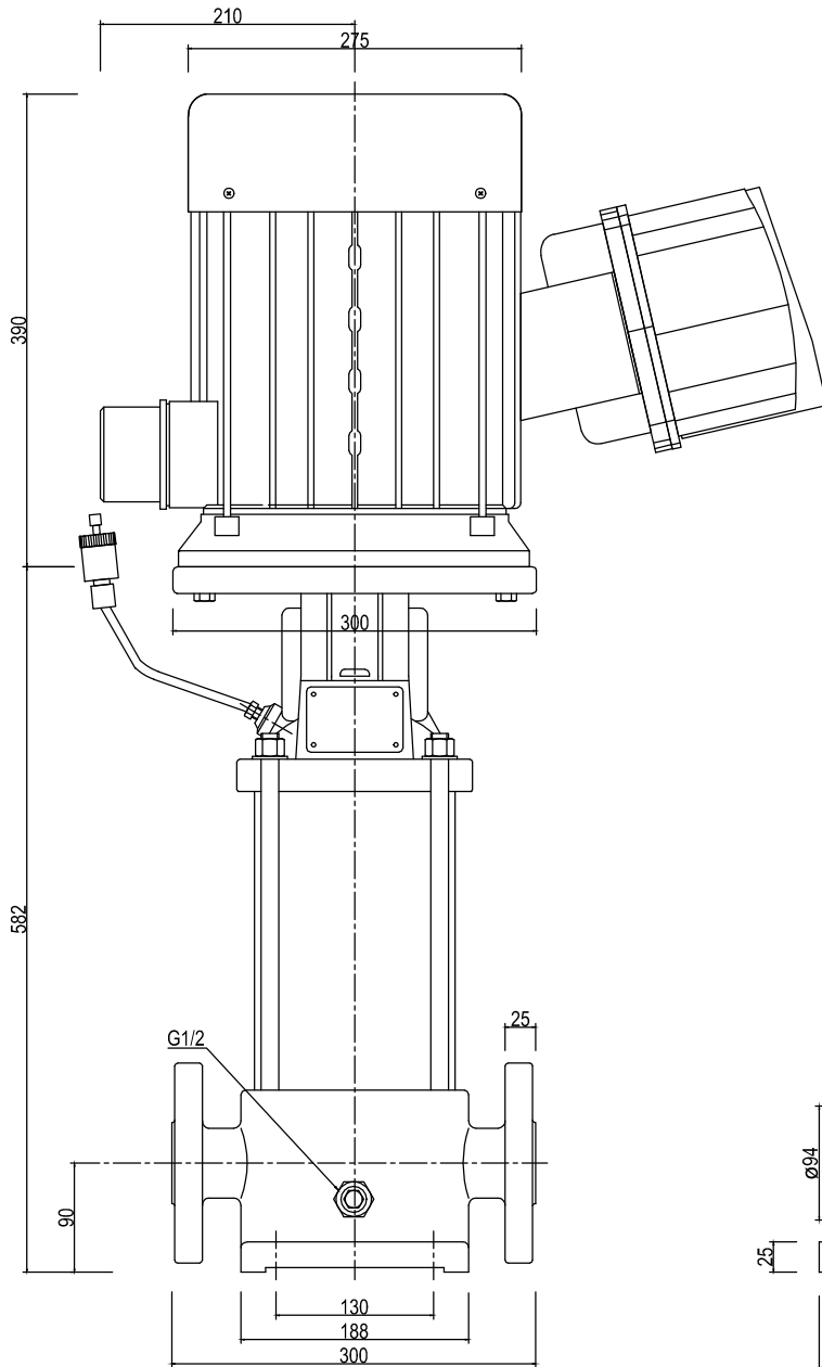
FGJ(DIN-ANSI-JIS) PN16-25-40(DN50) /mm/
