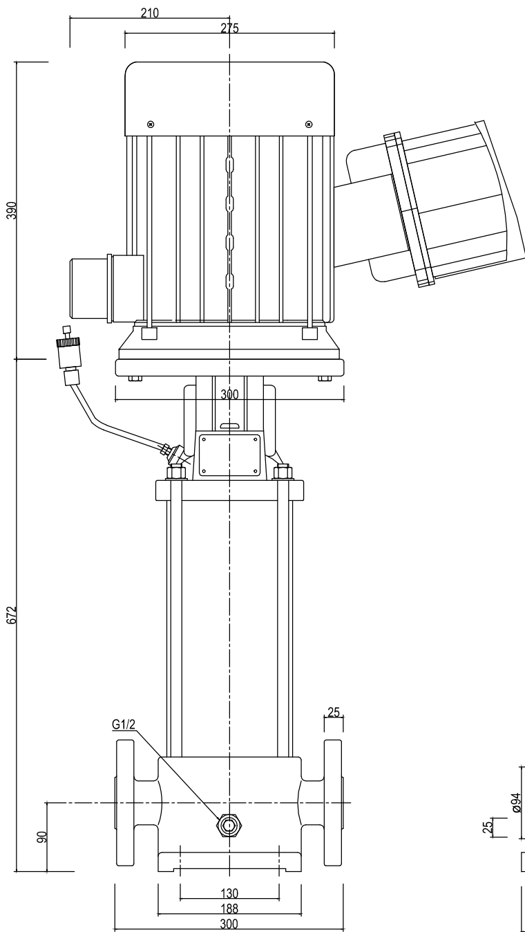
FGJ(DIN-ANSI-JIS) PN16-25-40(DN50) /mm/
